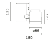
1x 35W CDM-TM
