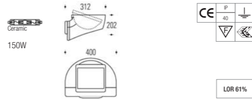
1x 150W CDM-TD RX7s Metal Halide
